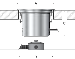
In-grade luminaire · Wall washer
