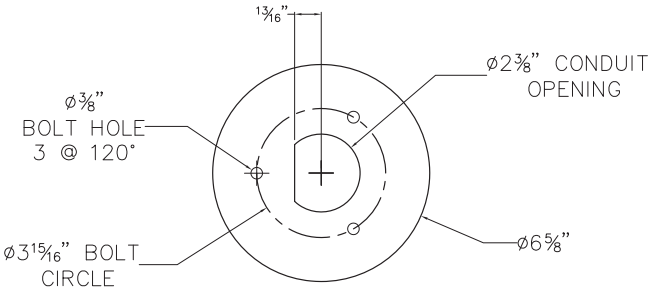
79 817 ANCHOR TEMPLATE
