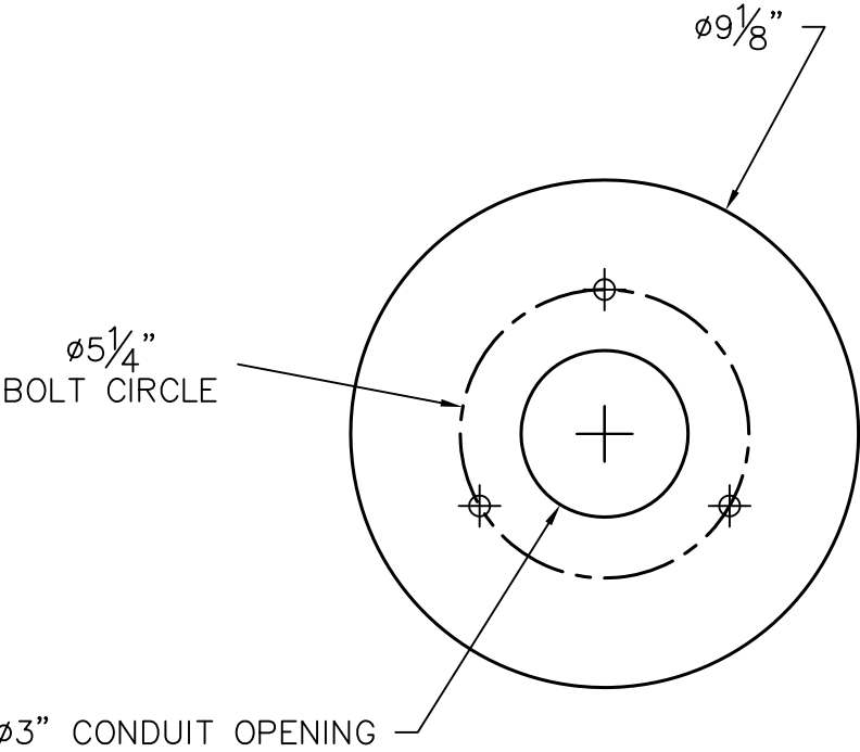
79 818 ANCHOR TEMPLATE
