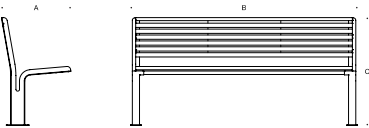
Bench · 14-slat
